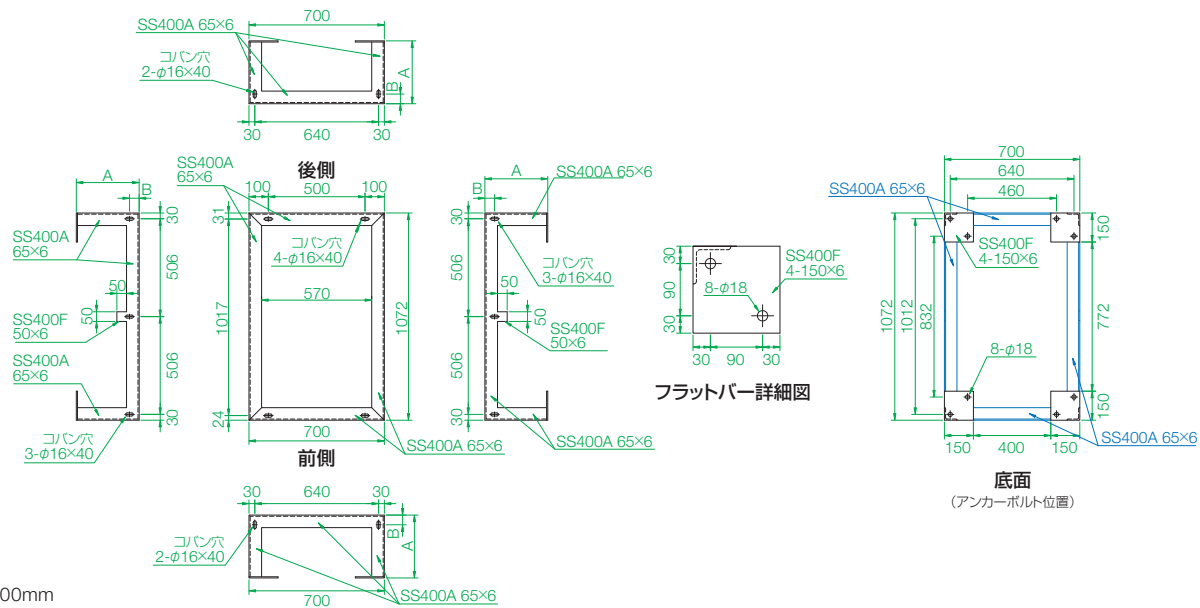
NetShelter SX 700標準架台 AR3130
