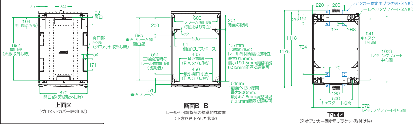
上面図 & 断面図 & 下面図
